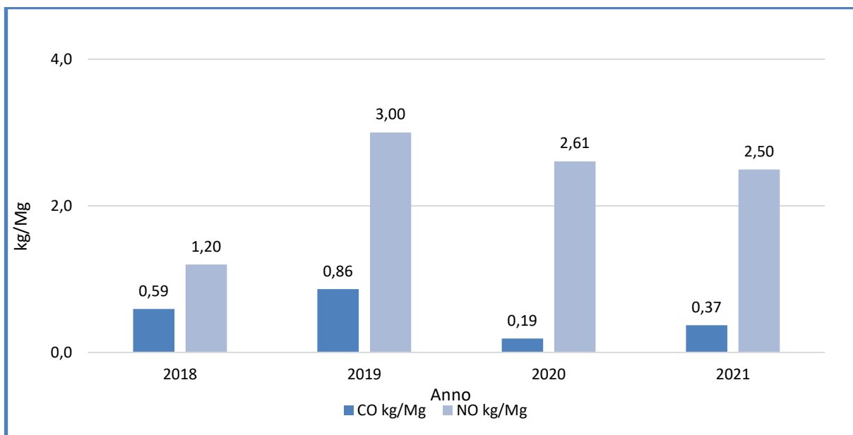
Grafico 10 kg di CO e NO emessi annualmente in rapporto alle tonnellate di rifiuti pirotrattati
