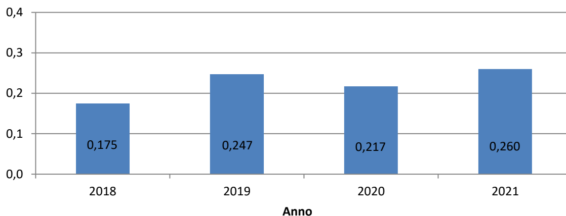
Grafico 9 Rapporto in peso tra reagenti chimici acquistati e rifiuti inviati al trattamento chimico/fisico
